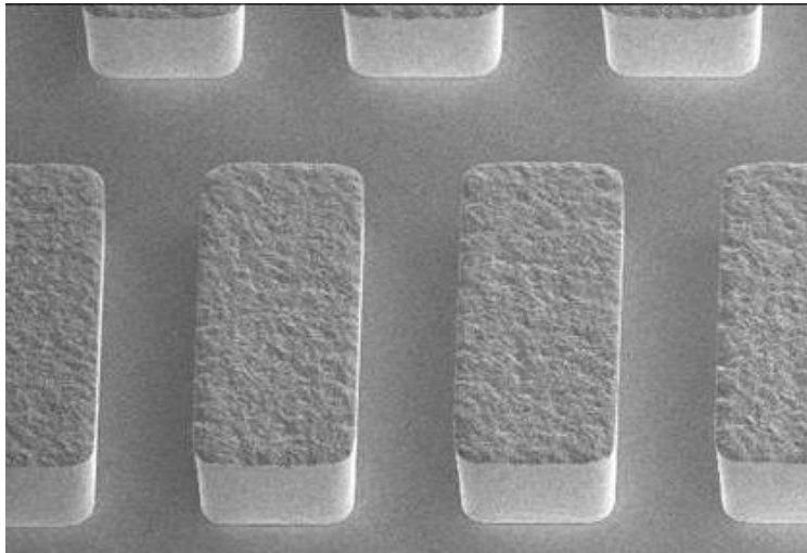
经无氰镀金液处理后的晶圆凸块形状实例（宽 30\mu\text{m} ）
