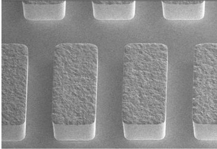
비시안 금도금액에 의한 웨이퍼 범프 형상 예(폭 30μm)
