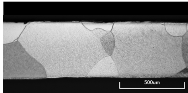
一般所使用的高純度白金之熱電偶導線
