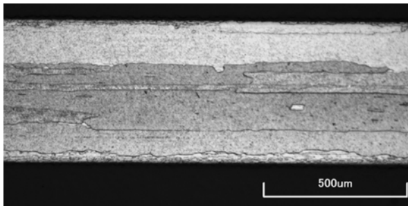
本次利用 ODS 白金開發成功的熱電偶線
