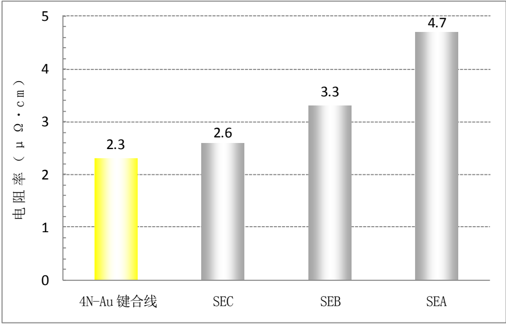
■电阻率的比较
