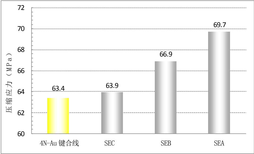
■在 FAB 压缩测试中硬度的比较
