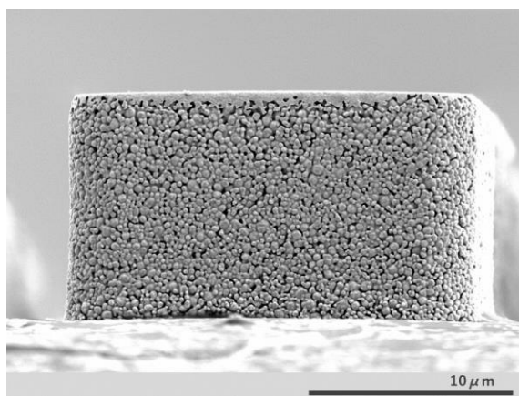
<AuRoFUSE™预制件的侧面 SEM 图像>
