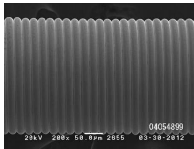
铂钨合金超细弹簧圈材料
